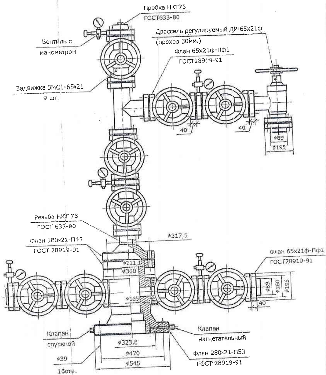
Рисунок 1. Арматура фонтанная АФК2-65*21
